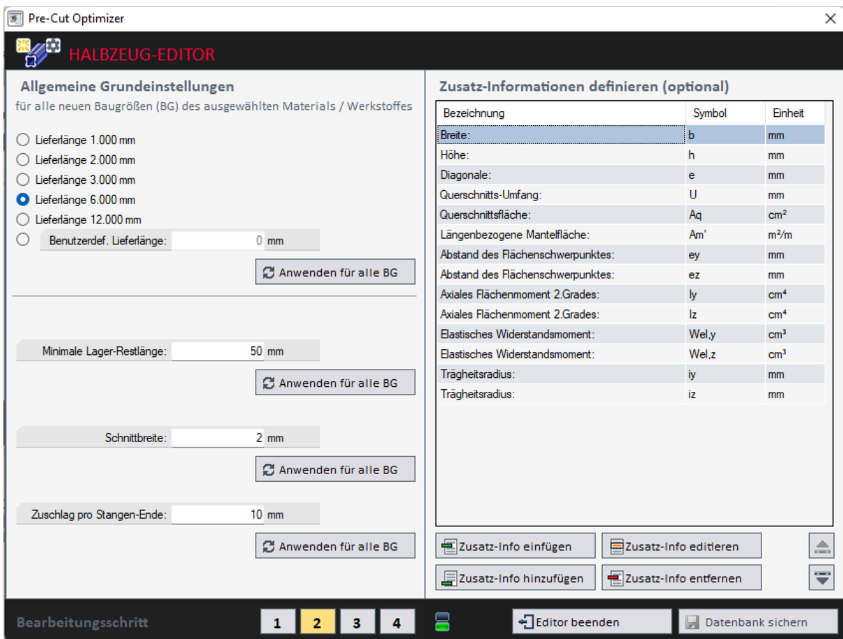
Bild 3-3: Halbzeug-Editor – Bearbeitungsschritt 2
